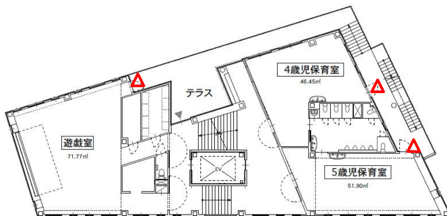
2階平面図
